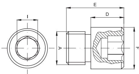
Perno Tipo: SECX..AQM
